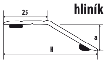
hliník
